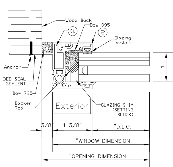
B JAMB Frame Depth: 1.625
