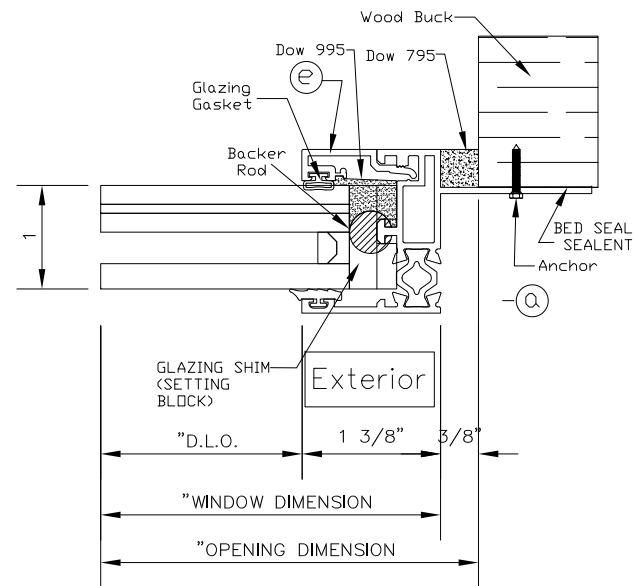
E JAMB Frame Depth: 1.625
